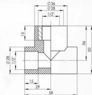
TEŠTIK SA UNUTAŠNJIM NAVOJEM TEE FEMALE THREADED
