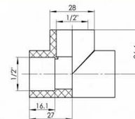
TEŠTIK / TEE
