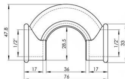
ZAobilazni luk duži LONG BRIDGE
