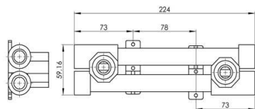
SET ZA BATERIJU SA SPOLJAŠNJIM NAVOJEM SHOWER VALVE BODY - MALE
