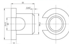
ROZETNA / ROSETTE
