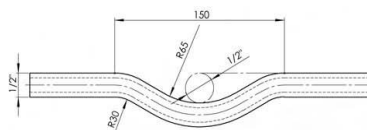
ZAobilazni luk duži LONG BRIDGE
