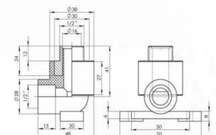
TEŠTIK SA UNUTAŠNJIM NAVOJEM TEE FEMALE THREADED
