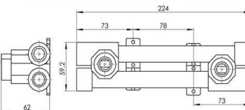
MUF SA ISPUSTOM SOCKET WITH OUTLET
