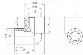
KOLENO SA SPOLJAŠNJIM NAVOJEM ELBOW - MALE THREADED
