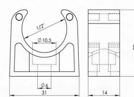
ŠELNA / PIPE CLAMP
