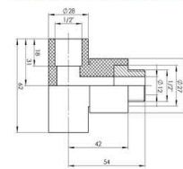
KOLENO SA UNUTAŠNJIM NAVOJEM ELBOW - FEMALE THREADED
