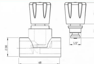
VENTIL SA UKRASNOM KAPOM VALVE WITH DECORATIVE KNOB
