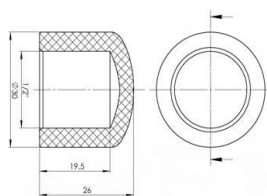
ČEP SA NAVOJEM / THREADED CAP
