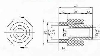
NIPLI SA SPOLJAŠNJIM NAVOJEM NIPPLE ROUND MALE
