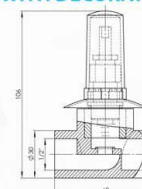
VENTIL SA UKRASNOM KAPOM VALVE WITH DECORATIVE KNOB
