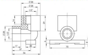
ZAVRŠNO KOLENO SA SPOLJAŠNJIM NAVOJEM END ELBOW - MALE THREADED
