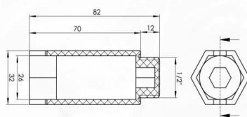
ČEP NAVOJ DUŽI / LONG THREADED CAP
