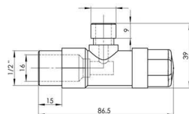
PRIKLUČAK ZA VEŠ MAŠINU WASHING MACHINE CONNECTION
