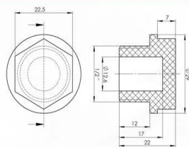
ČEP NAVOJ DUŽI / LONG THREADED CAP
